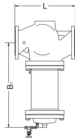
VFQ D_y 150 - 250 с удлиненным штоком для t > 150\text{ }^\circ\text{C}
